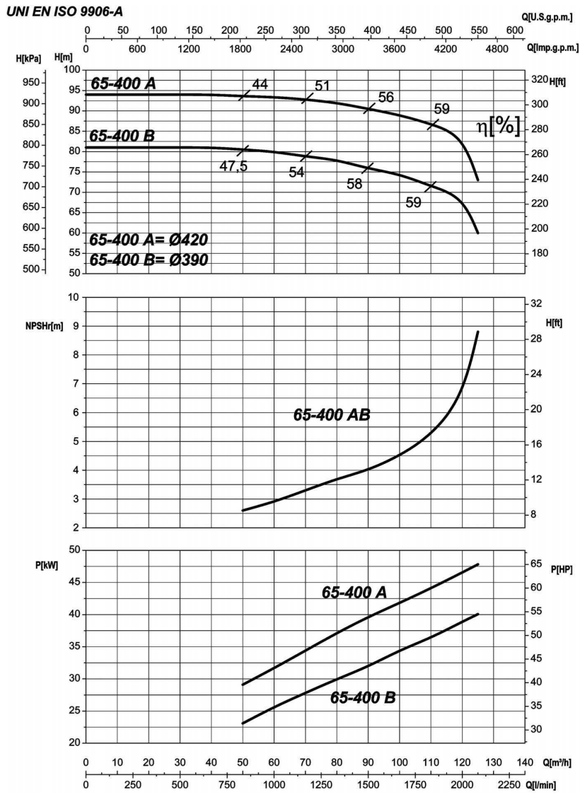
65-400 6NCBZ4P / NCB
