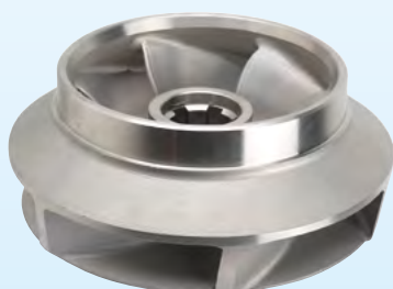
PRECISION CAST STAINLESS STEEL AISI 316 IMPELLERS GIRANTI IN AISI 316 MICROFUSO IMPULSORES DE ACERO INOXIDABLE MICROFUNDIDO AISI 316
