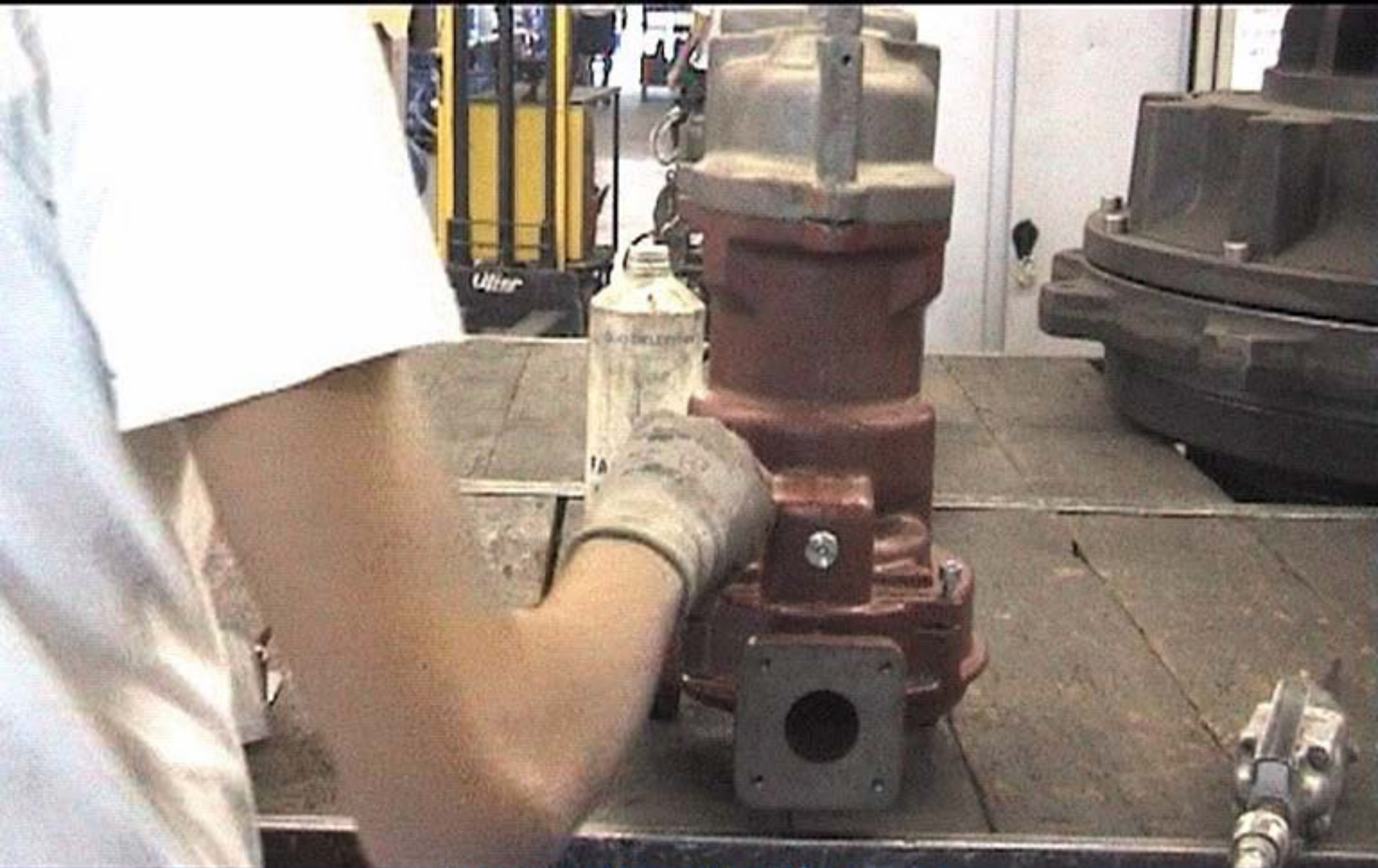
Serraggio viti diffusore Screw locking of the pump body
